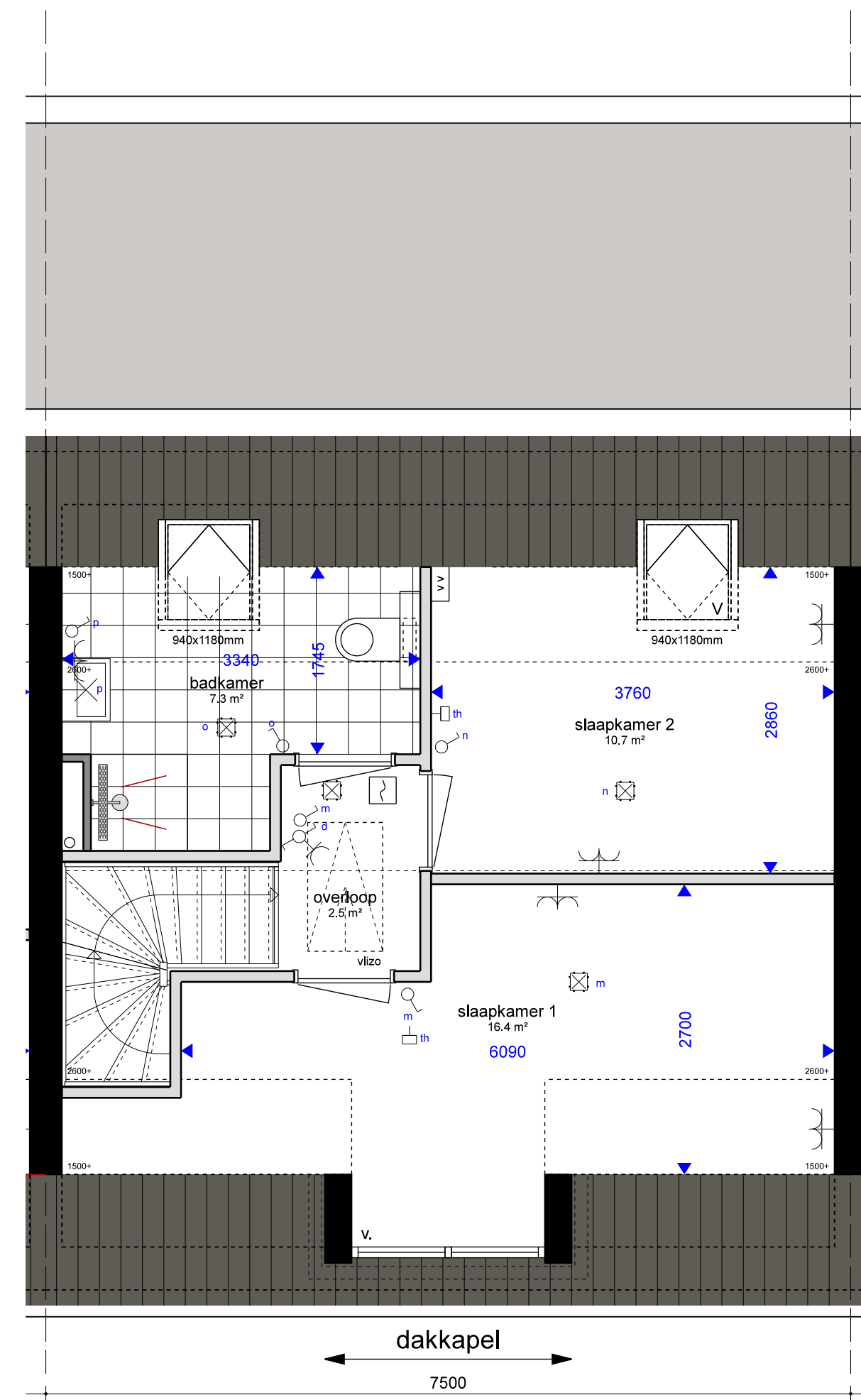
VERDIEPING
