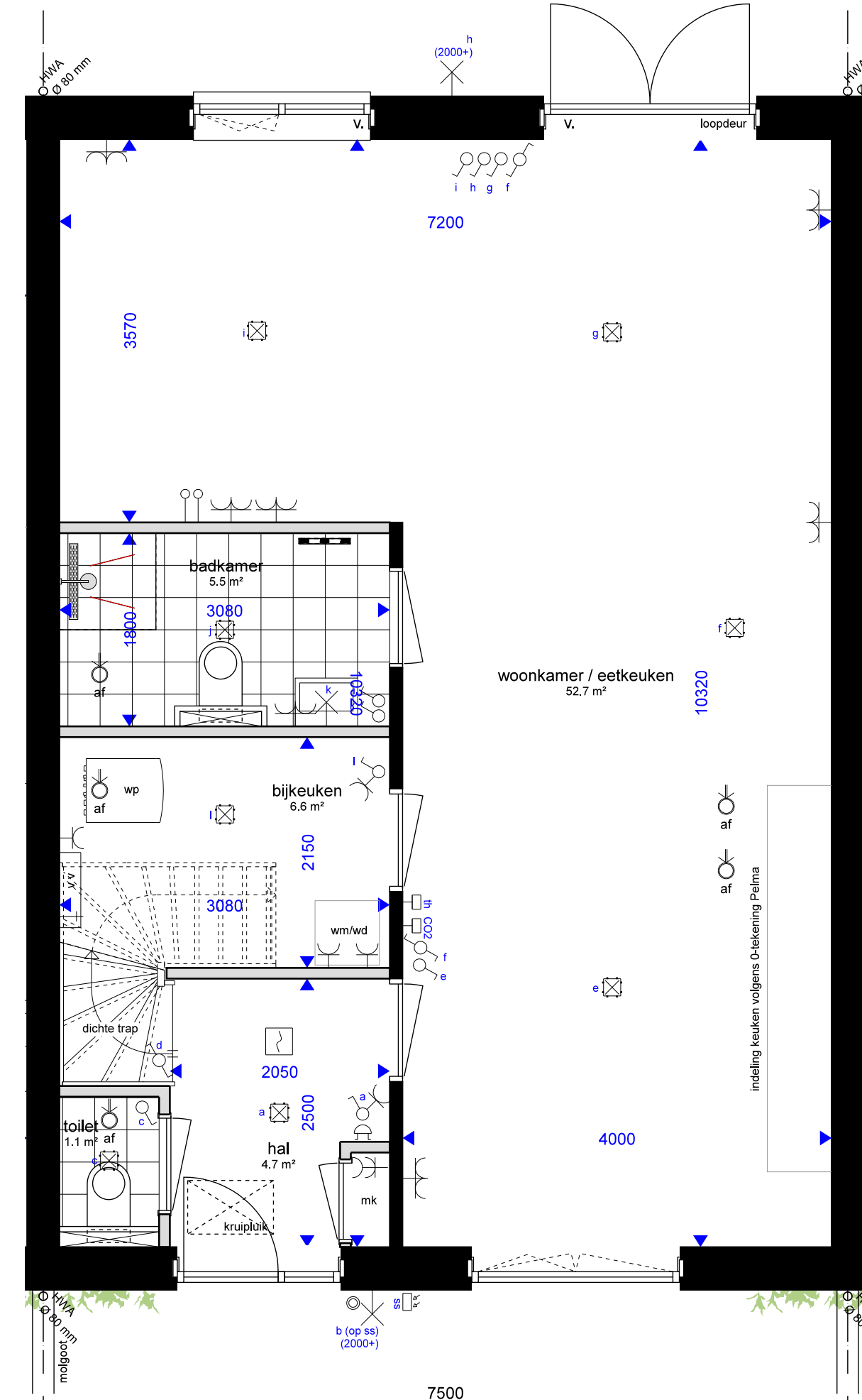
BEGANE GROND
