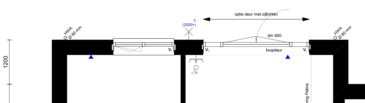
BEGANE GROND
